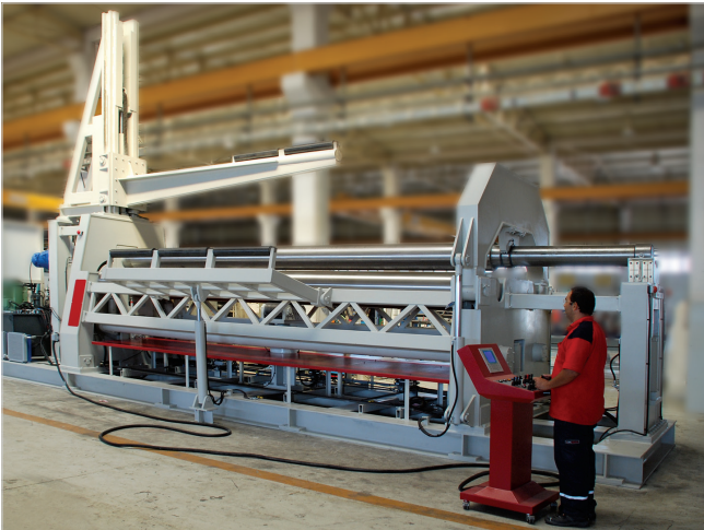
Pre-stress plate bending machine for tube bending Boru üretimi için ön gerilmeli özel silindir makinesi
