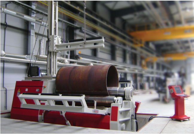
AHK 25-10
