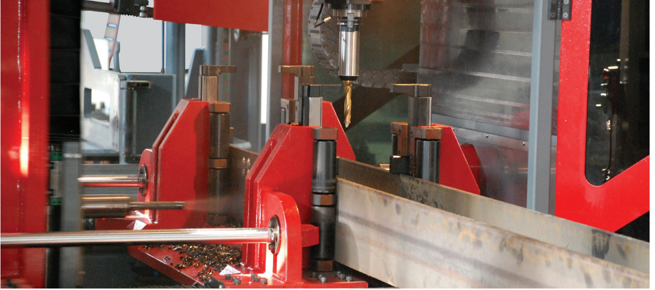
Aynı bağımsız spindle ünitesi sayesinde profilin üç tarafına aynı anda delik delinebilir
